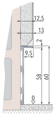
Plintă instalată pe perete din zidărie Profil 13 mm
