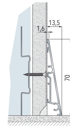
Plintă instalată pe perete din gips carton (simpla placare din gips carton)
