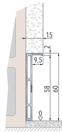
Plintă instalată pe perete din zidărie Profil 15 mm
