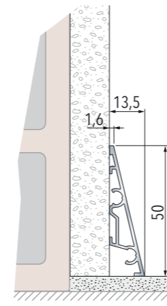
Plintă instalată pe perete din zidărie
