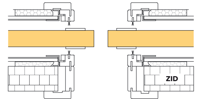
Versiune cu captuseala de perete
