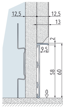
Plintă instalată pe perete din gips carton (2 plăci de gips-carton) Profil 13 mm
