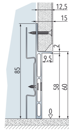
Plintă instalată pe perete din gips carton (o placă din gips carton) Profil 15 mm
