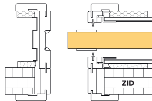
Versiune cu captuseala de perete
