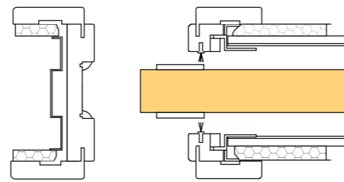
Versiune fara captuseala de perete
