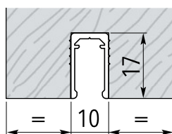
Detaliu panou de ușă cu profil Security
