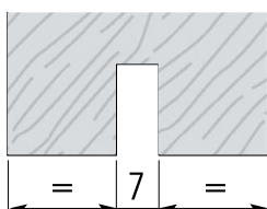
Detaliu panou de ușă cu ghidaj de ușă standard (doar frezat)
